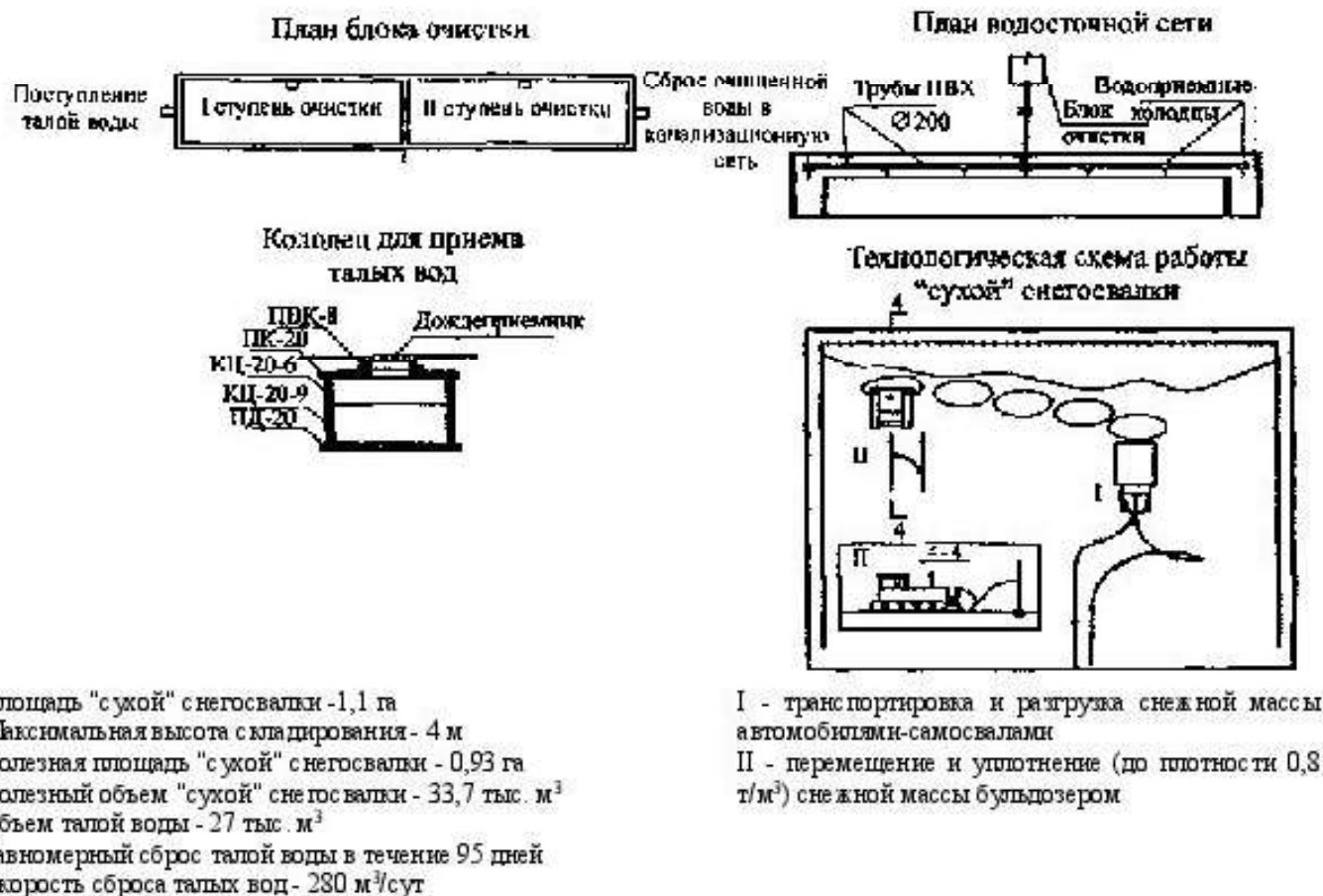
Рисунок 5.1 – Схема «сухой» снегосвалки
